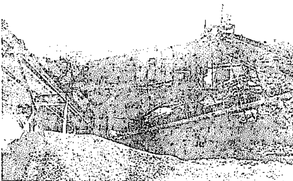
Foto 2. Zaranda clasificadora de piedra caliza.
